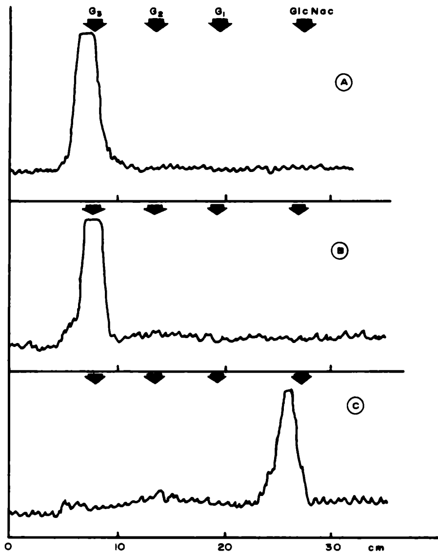
Fig. 26 - Estudio de la acción de la \beta -N-acetilglucosaminidasa sobre X_3 . (este compuesto está marcado en la GlcNac del extremo reductor). A= control incubado sin enzima; B= X_3 incubado con enzima obtenida de saliva humana; (dador M Tabla V). C= X_3 incubado con la glicosidasa purificada de oviducto de gallina.
