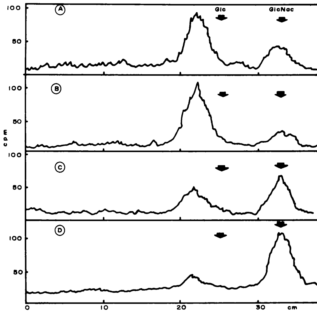
Fig. 17 - Estudio del efecto del pH en la formación del lípi- do-disacárido .
