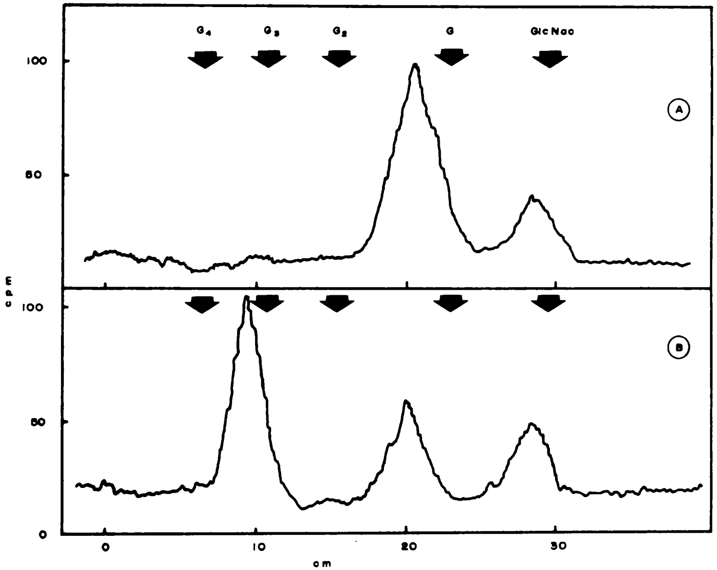
Fig.19 - Perfil cromatográfico de los productos de hidrólisis ácida suave del lípido-azúcar formado por la incubación de dol-P-P-(GlcNac) 2 -radioactivo y GDP-Man no marcado. A=control B=incubación con preparaciones enzimáticas de oviducto de gallina.
