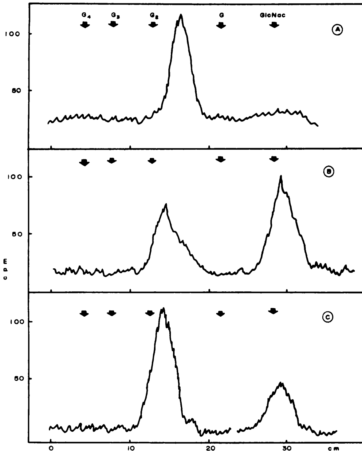
Fig. 14 - Acción de \beta -N-acetilglucosaminidasa sobre la di-N-acetilquitobiosas.
