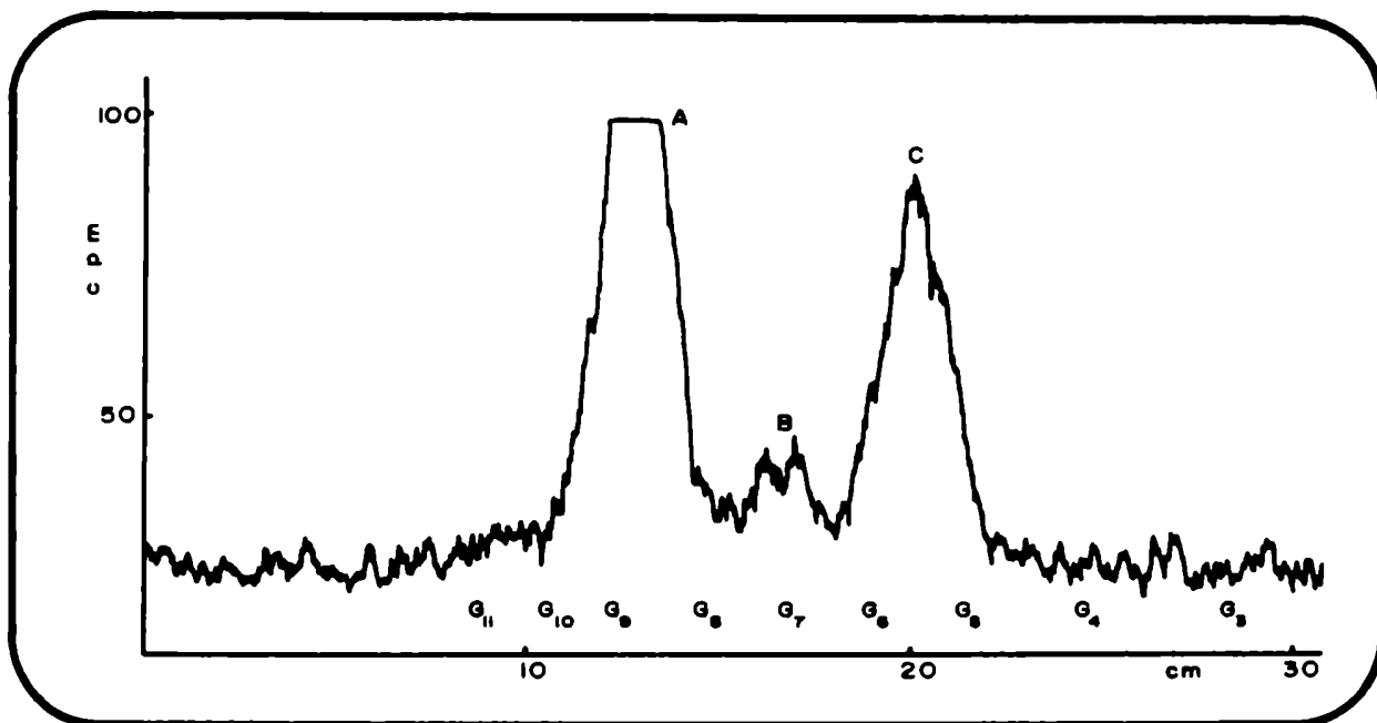
Fig. 31 - Perfil de cromatografía en papel del oligosacárido sintetizado a partir del lípido- \chi_3 y dolicol-P-Ma_nosa.
