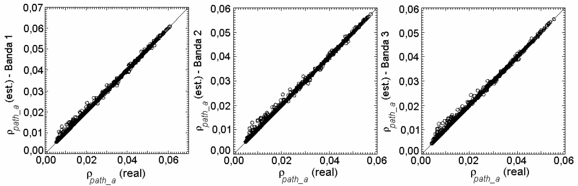
Figura 3.15 Regresión lineal entre la reflectancia debida a los aerosoles estimada y real para cada una de las bandas del VIS del sensor MMRS (1, 2 y 3).
