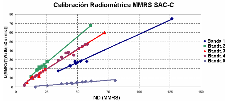
Figura 3.17 Radiancia (L) del sensor MMRS en función del número digital (ND). Ajuste lineal para cada banda ( r^2 > 0,95 ) luego de la calibración cruzada entre el sensor MMRS y el Landsat 7 ETM+ (modificado Bratina et al. 2003).
