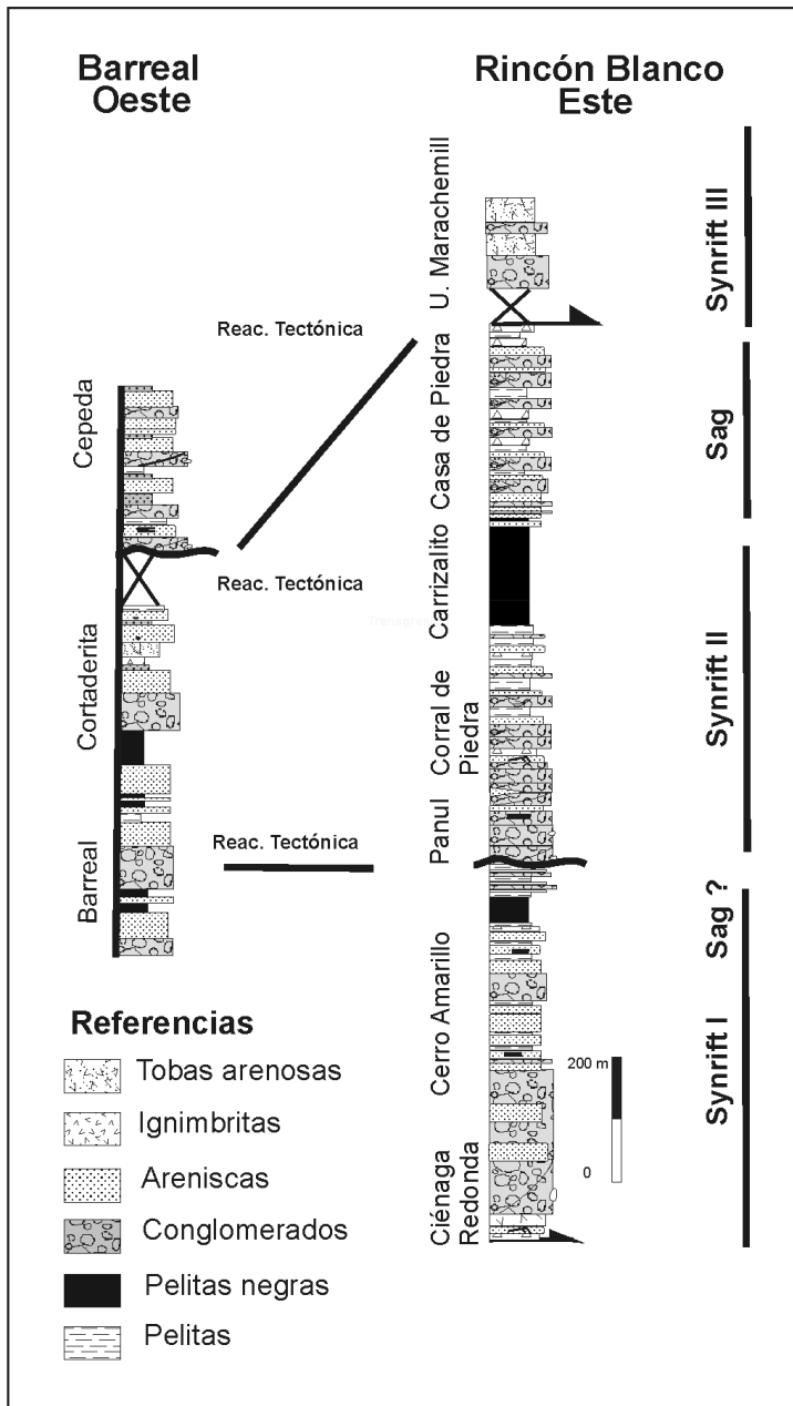
Figura 6: Correlación preliminar entre la Unidad Marachemill y la Formación Cepeda, basada en los trabajos realizados hasta el momento por Bonati et al. (2008). Como puede observarse hay una buena correspondencia entre ambas unidades desde el punto de vista tectonoestratigráfico.
