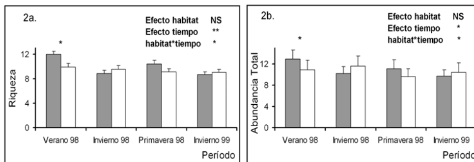
FIG. 2. Promedios y error estándar para: a) riqueza (número de especies), y b) la abundancia total (individuos por 10 min de conteo) para el bosque (barras grises) y para el desarbastado (barras blancas), durante el verano (Marzo 1998), la primavera (Diciembre 1998) y el invierno (Agosto 1998 y 1999) en la Estación Experimental “La María”, Provincia de Santiago del Estero, Argentina. Se indican los resultados del ANOVA de dos factores con medidas repetidas en un factor (tiempo) y, cuando corresponde, se indica la estación donde se registró la interacción (* = P < 0.05 ; ** = P < 0.01 ).
