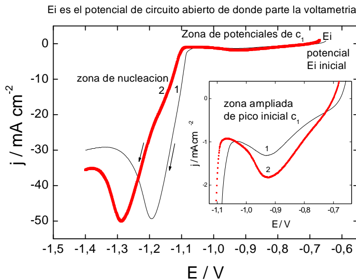
Figura 1.1.a. Depósito voltamétrico de cinc a partir de soluciones de electrodeposición a: ( \text{NH}_4\text{Cl} 1,6 M + \text{Zn Cl}_2 0,3M) y solución b: ( \text{NH}_4 ) 2 \text{SO}_4 1,3M \text{ZnSO}_4 0,3M). Potencial de partida E_i . voltametría 1- solución a: 100%. Voltametría 2- solución b: 100%. b. Ampliación en la zona de potenciales de c_1 a partir de cloruros ó de sulfatos. Velocidad de barrido 10 \text{ mV s}^{-1} . pH 4, I = 2,5\text{M} .
