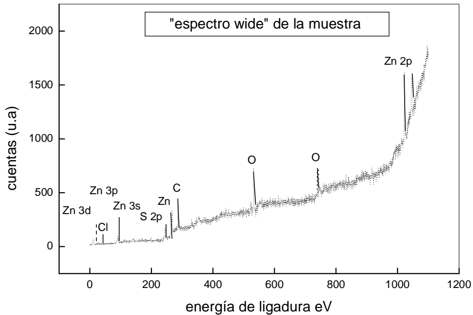
Figura 1.6. Espectro amplio "Wide" ó amplio en energía de la muestra.
