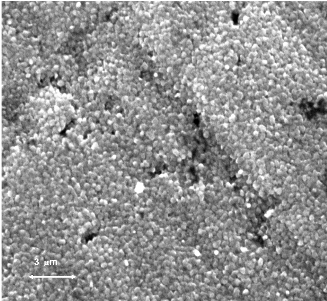
Figura 1.5. Fotomicrografía obtenida por SEM en depósitos (a) medio de sulfatos. Se utilizó la técnica voltamétrica seguida de potenciostática en la zona de control activado. Voltamétrica desde E_i = -0,5.6V hasta I_g < 100 \mu Acm^{-2} , luego el barrido a 100 mV s^{-1} hasta E_g , seguido de deposición potenciostática en E_g -1,14 V , durante 100 s. Solución de electrodeposición: (NH_4)_2SO_4 1,3M + ZnSO_4 0,3M. Zona analizada 1mmx1mm. 10000X.
